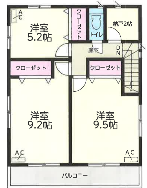
2階平面図:54.67㎡
