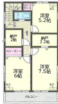
2階平面図:48.60㎡
