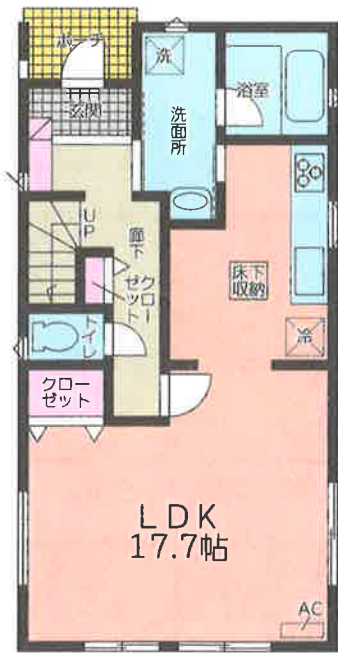
1階平面図:47.38㎡
