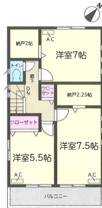
2階平面図:48.60㎡
