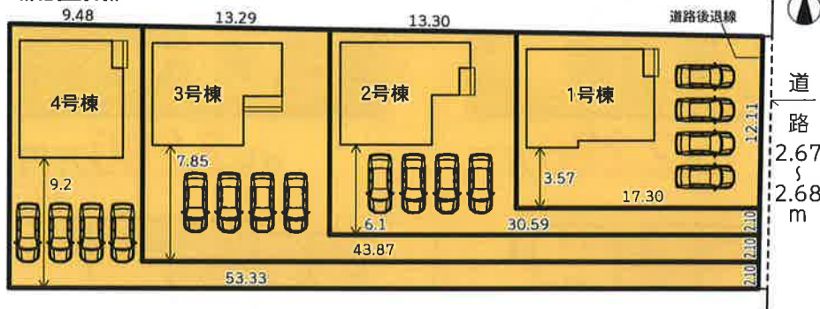
《配置図》
