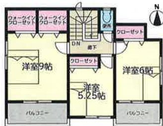
2階平面図:48.85㎡(14.77坪)
