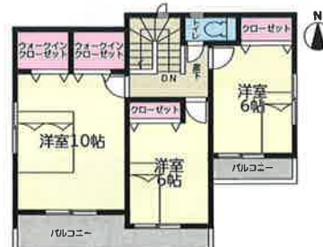
2階平面図:52.58㎡(15.90坪)
