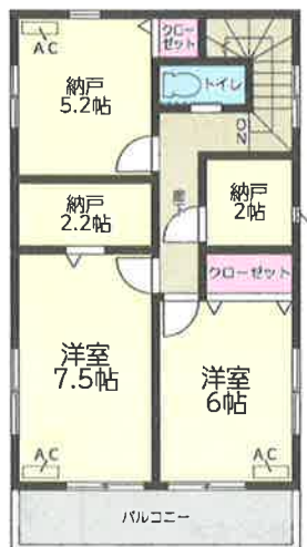
2階平面図: 48.60㎡
