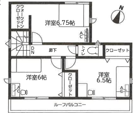
2階平面図:44.72㎡
