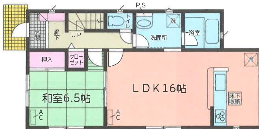
1階平面図:55.08㎡
