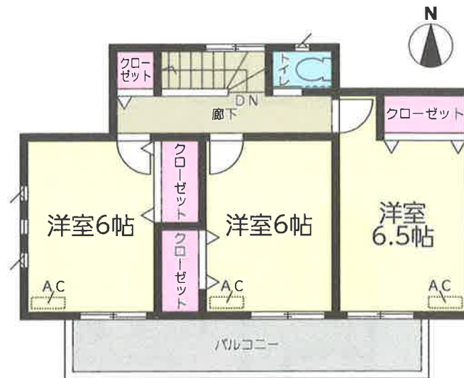
2階平面図:42.93㎡
