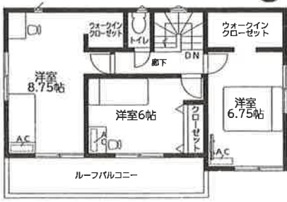
2階平面図:49.07㎡
