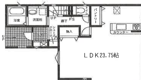
1階平面図:60.86m 2
