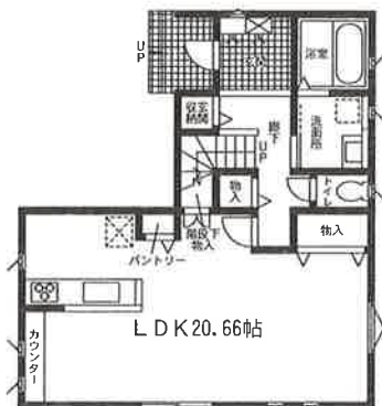
1階平面図:56.31m 2
