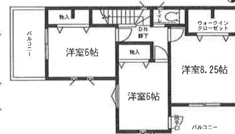
2階平面図:48.85m 2
