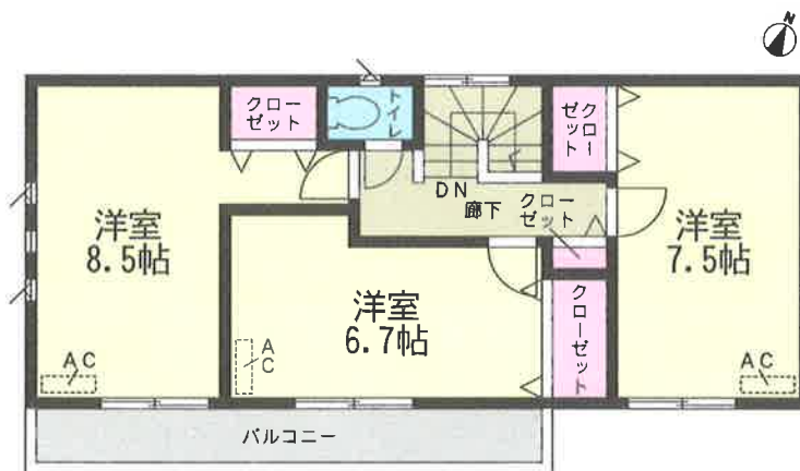
2階平面図: 48.60㎡
