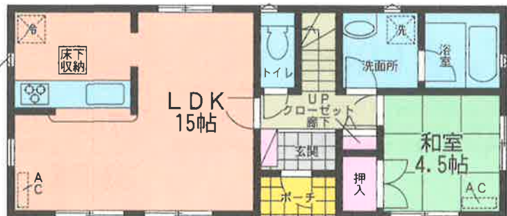
1階平面図: 46.98㎡
