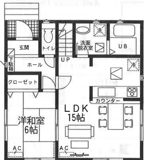
1階平面図: 51.35m 2
