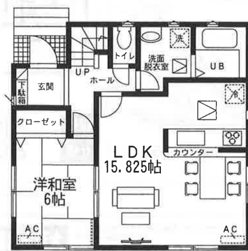
1階平面図: 53.83m 2
