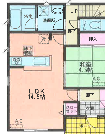
1階平面図:48.60m 2
