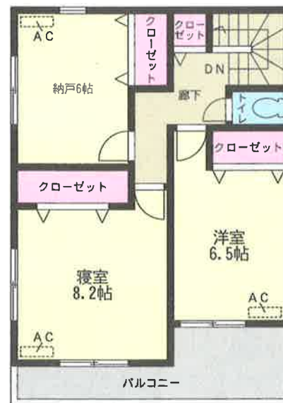
2階平面図:48.60m 2
