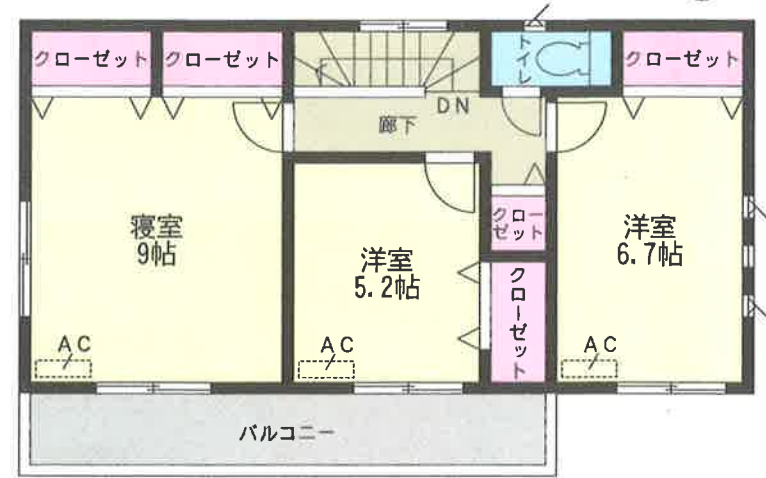
2階平面図: 49.00㎡
