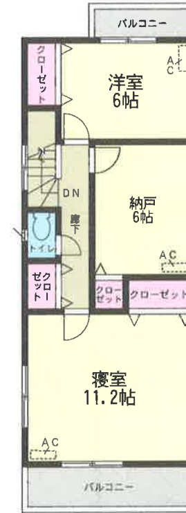
2階平面図: 50.62㎡
