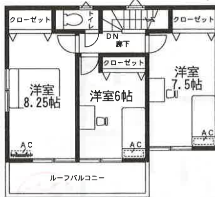
2階平面図: 47.21㎡
