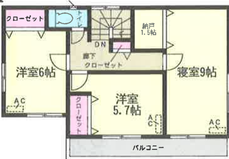
2階平面図: 48.60㎡
