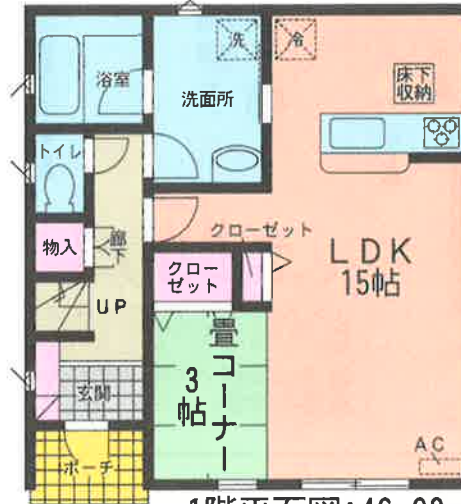
1階平面図:46.98㎡
