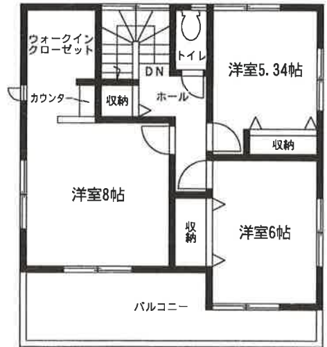
2階平面図: 48.86㎡
