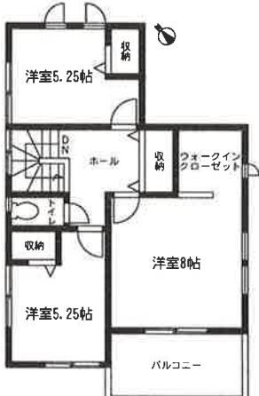
2階平面図：47.21㎡
