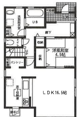
1階平面図：60.46㎡
