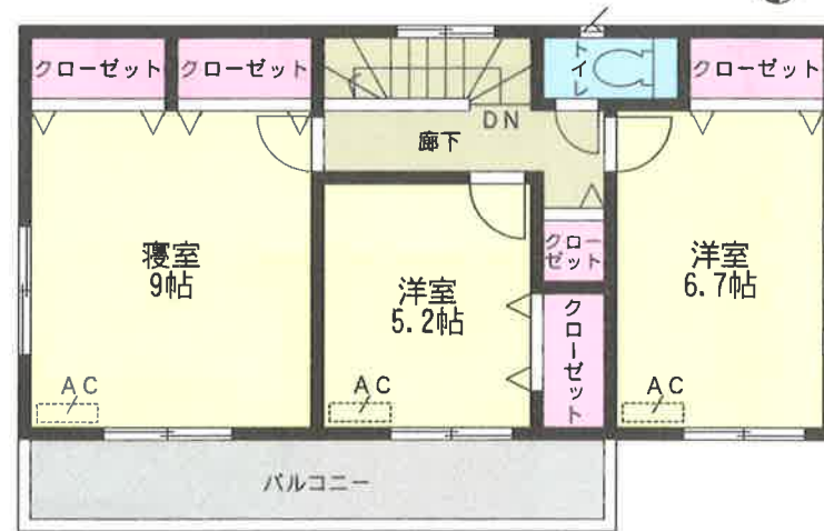
2階平面図: 49.00㎡
