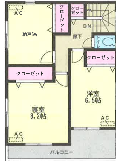
2階平面図: 48.60m 2
