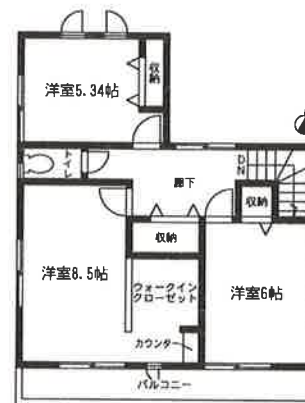
2階平面図：49.69㎡
