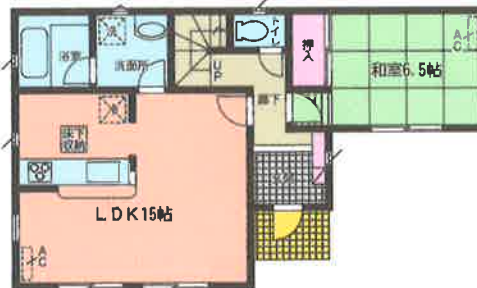
1階平面図: 51.84㎡
