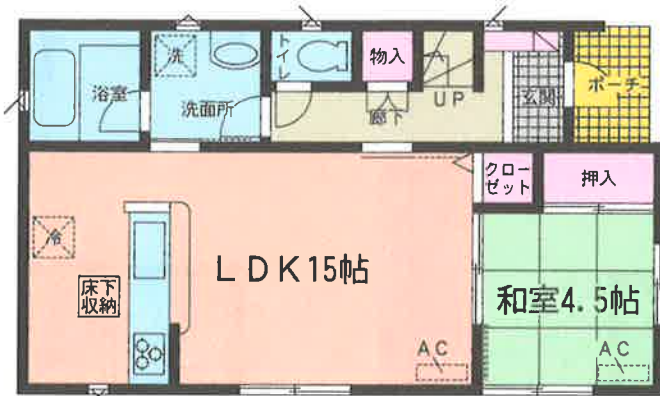
1階平面図: 48.60㎡
