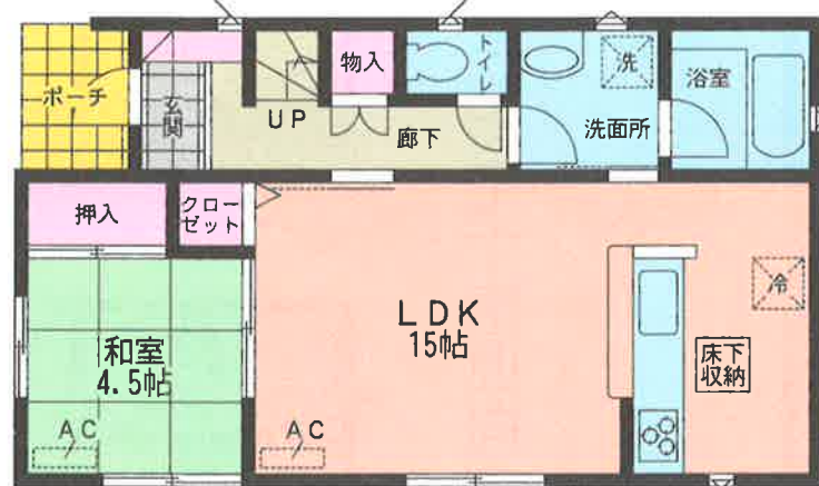
1階平面図: 48.60㎡
