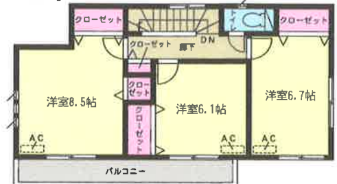
2階平面図:48.80㎡
